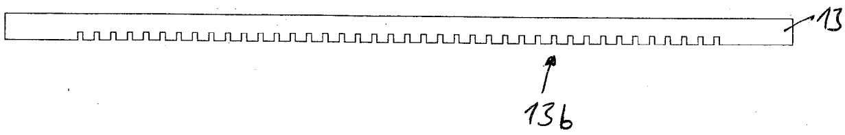
Fig. 4 Detail Kamm (2:1)
